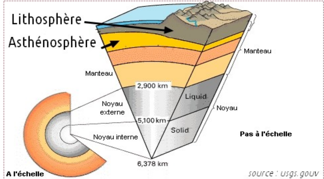
LA STRUCTURE DU GLOBE
