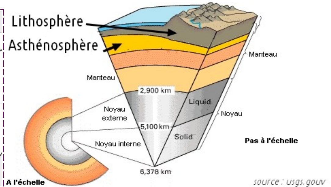
LA STRUCTURE DU GLOBE
